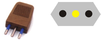
Tipo L Italia 10A
